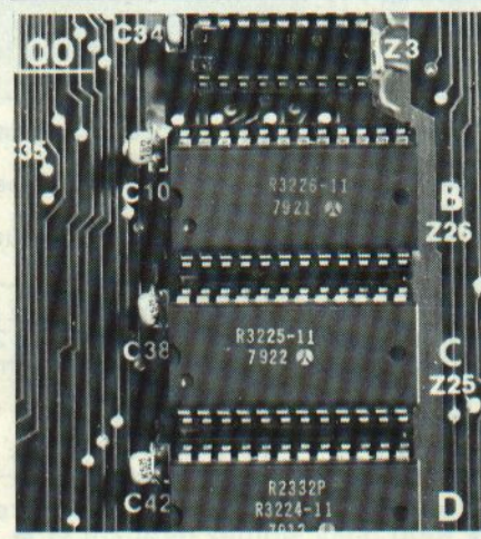
Gros plan sur les mémoires : les MEV (en haut) voisinent avec les MEM BASIC (B et C) et assembleur (D).
